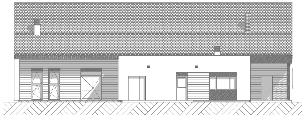
E-2 Elewacja tylna 1:200
