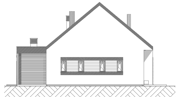
E-4 Elewacja boczna II 1:200
