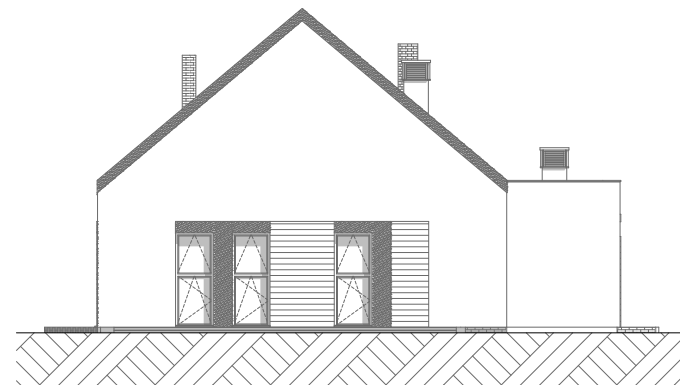
E-3 Elewacja boczna I 1:200
