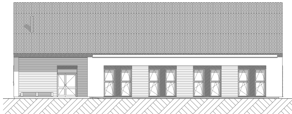
E-1 Elewacja frontowa 1:200
